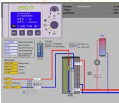
Visualisierung / E-Control
